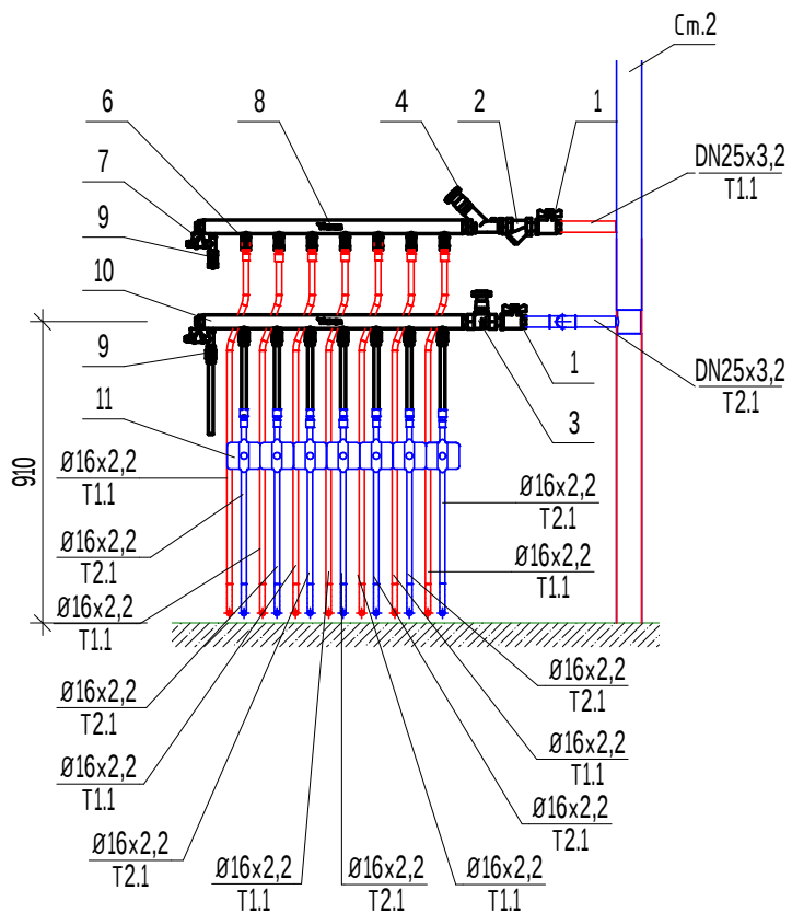
Коллектор на 7 выходов (16-27 этаж, Ст.2)
